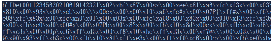
Fig. 13. Decrypted data.
